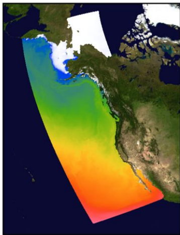
1980-04-01 sea surface temperature (°C)
